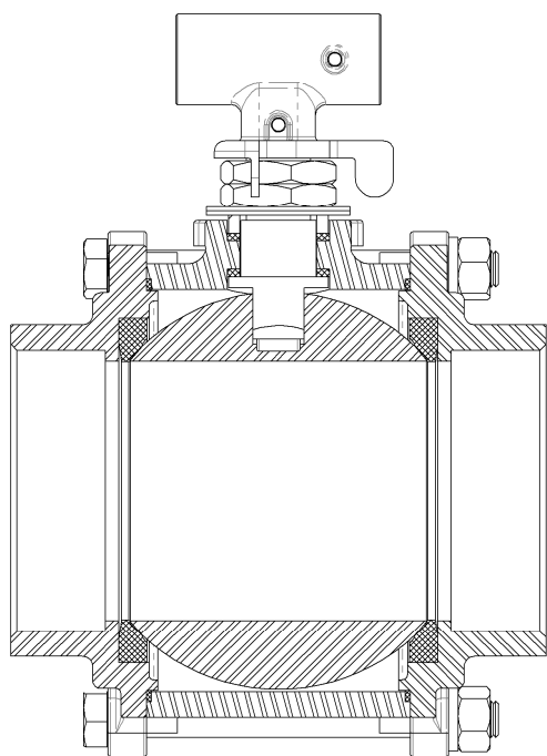
Figura 1 – Corte transversal da VET 4\"/>
